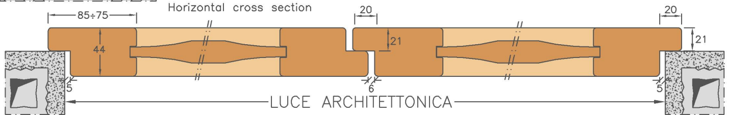
SEZIONE ORIZZONTALE Horizontal cross section
