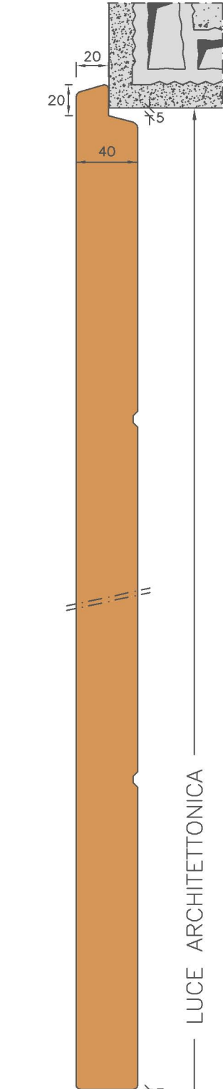
SEZIONE VERTICALE Vertical cross section
