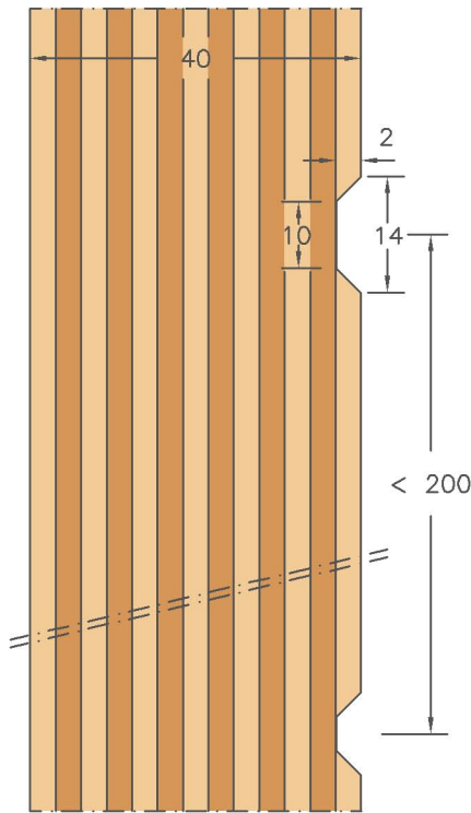
DETTAGLIO FRESATURA ORIZZONTALE Particular of horizontal milling
