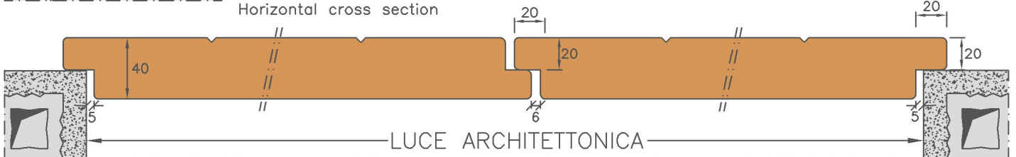
SEZIONE ORIZZONTALE Horizontal cross section
