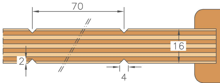
PROSPETTI INTERNO-ESTERNO Con fresature verticali Internal-external views
